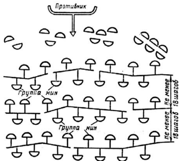
Стандартная схема миниурования, принятая в армиях стран НАТО
